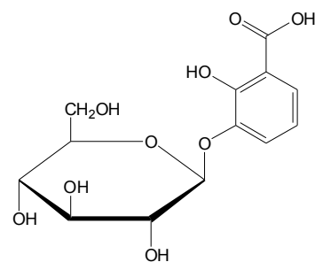
2,3-DHBAG
